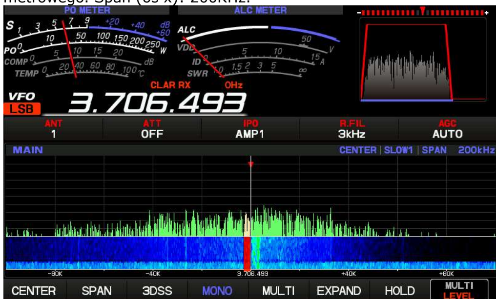
Preselektor włączony i dostrojony do częstotliwości pracy – 3706 KHz. Span: (oś x): 200KHz. Różnica wyraźna w stosunku do wykresu poprzedniego.
