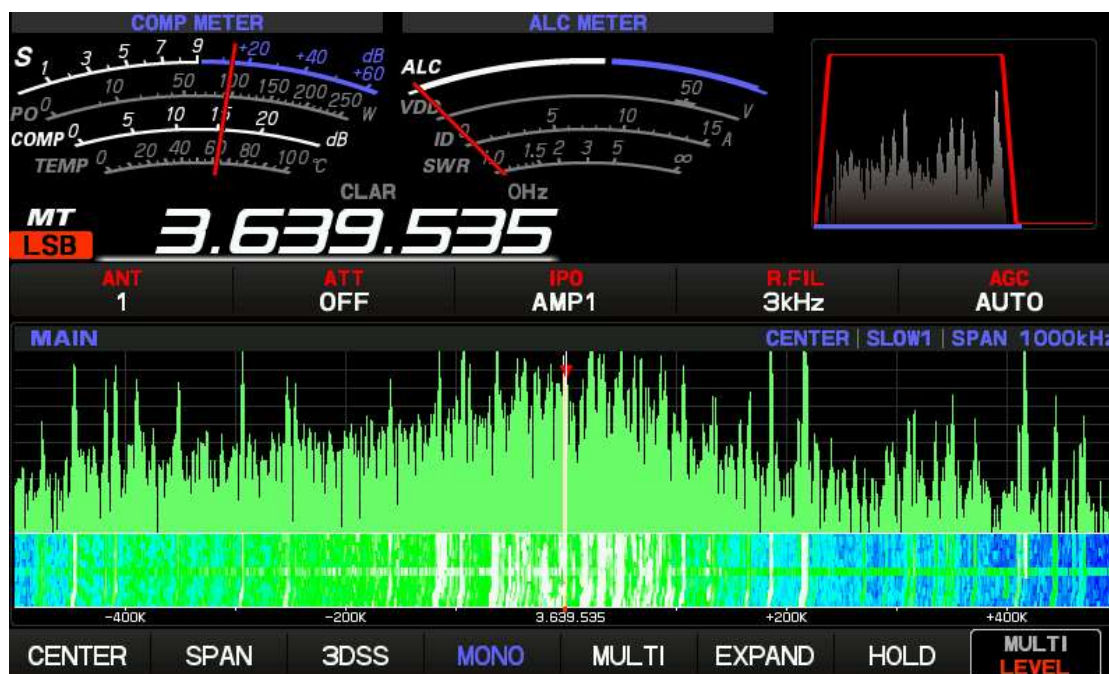
Foto-1. Preselektor włączony i dostrojony do częstotliwości pracy – 3639 KHz. Widać potężne sygnały, w tym zakłócające w pasmie 80-metrowym. Span (oś x): 1MHz.
