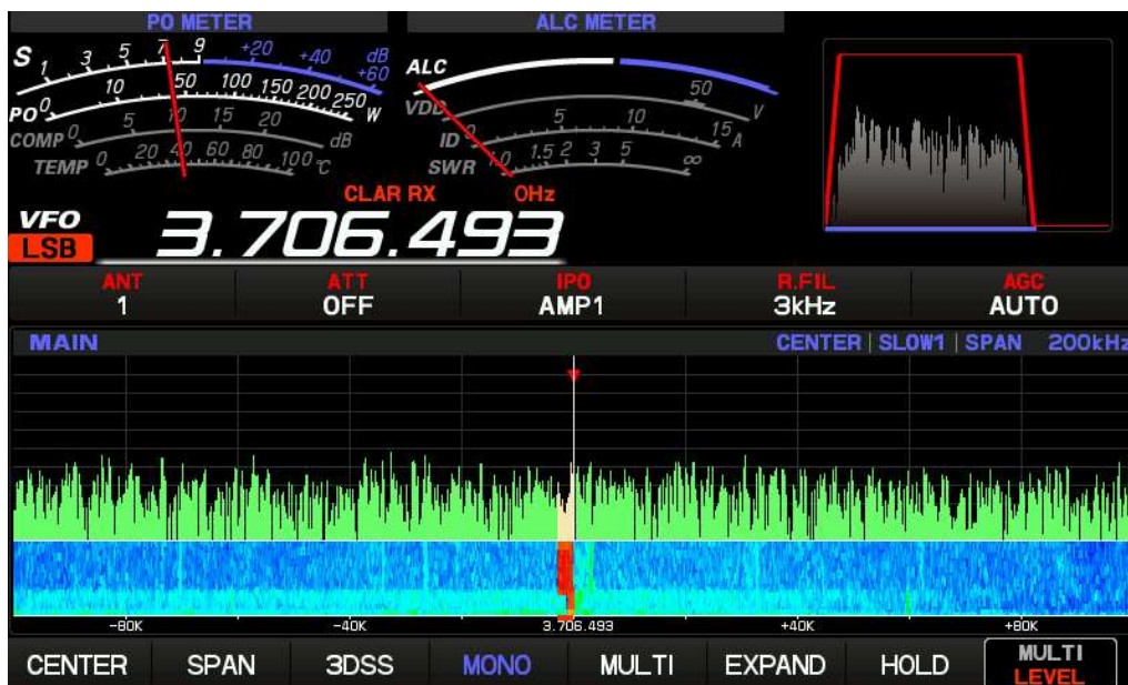
Foto-2. Preselektor wyłączony. Widoczna równomierna wartość szumu pasma 80-metrowego. Span (oś x): 200KHz.
